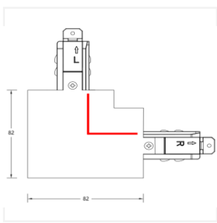
MT5-R563R L 型连接器
