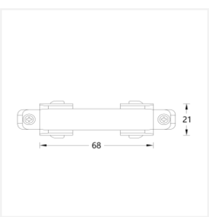
MT5-567 小 I 型连接器
