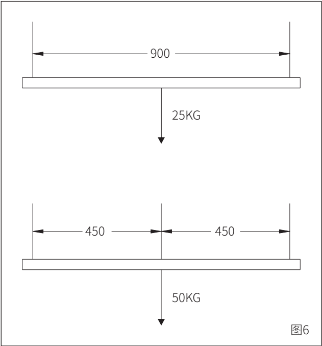
9.最大吊重示意图（图6）。
