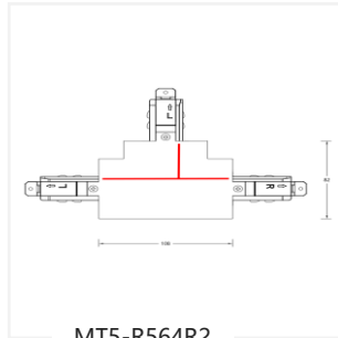
MT5-R564R2 T 型连接器
