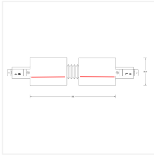
MT5-R569 软连接器
